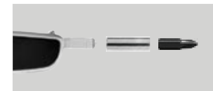
Bitadapter mit Bits zum Aufstecken auf den Glasbrecher
